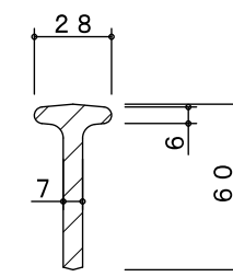
B-B断面図 S = 1/3
