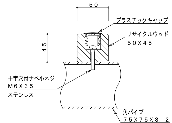
A詳細図 S=1/3
