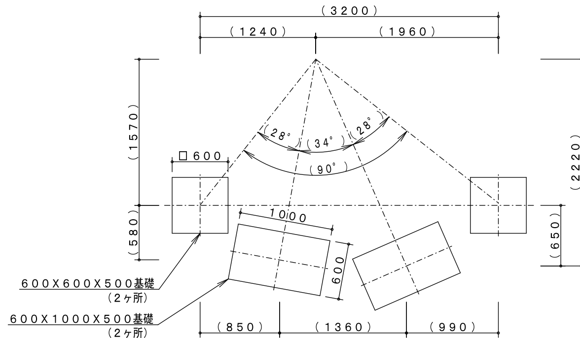
基礎平面図
