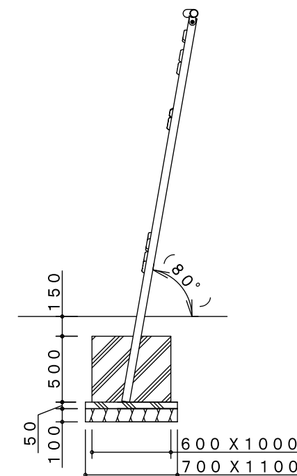
A-A矢視図
