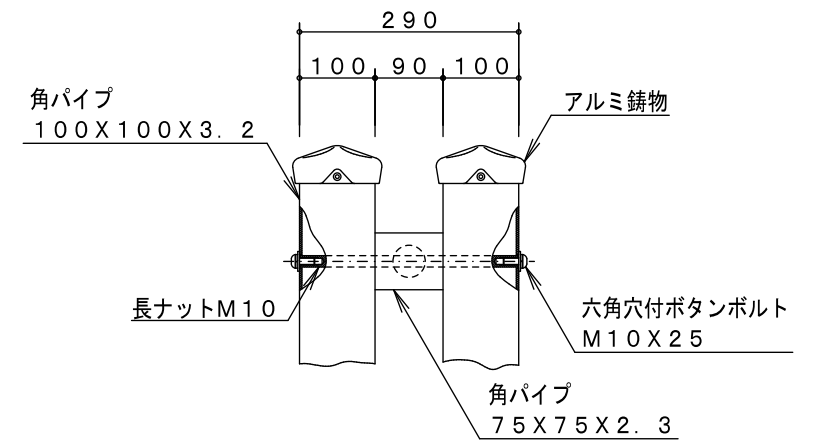
A 詳細図 S=1/10
