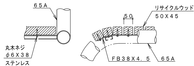
A詳細図 S=1/10
