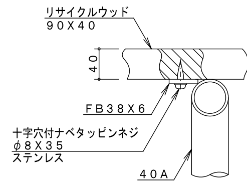
A詳細図 S=1/5
