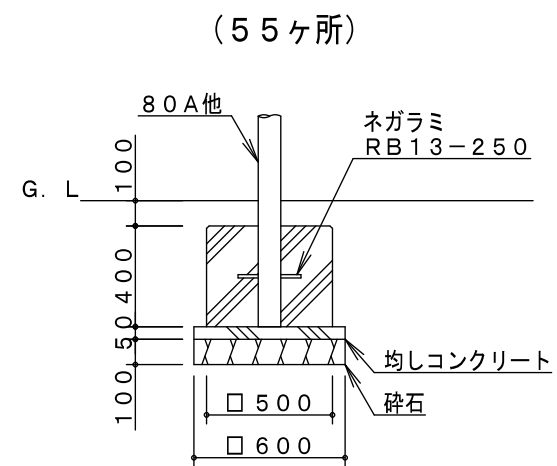
A基礎詳細図
