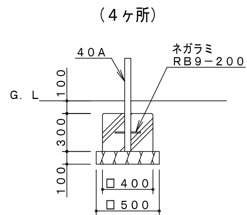
B基礎詳細図
