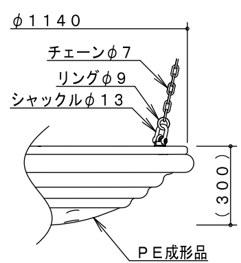
吊席 (C) 詳細図 S=1/20
