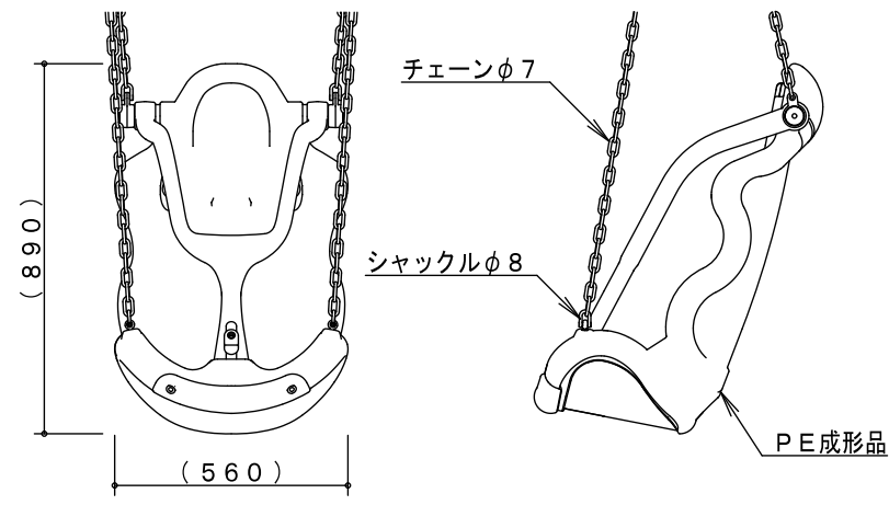
吊席 (A) 詳細図 S=1/20
