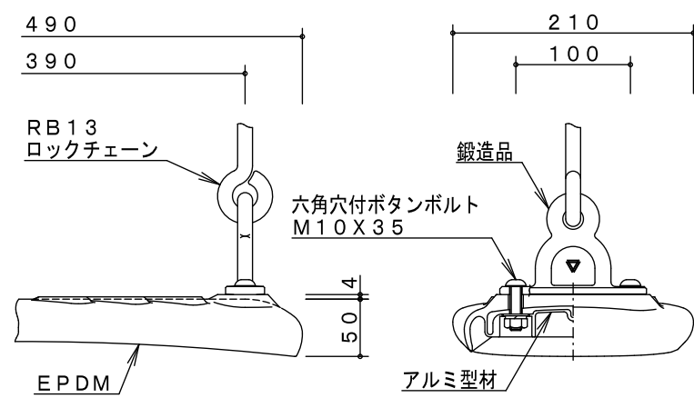
吊席 (B) 詳細図 S=1/6
