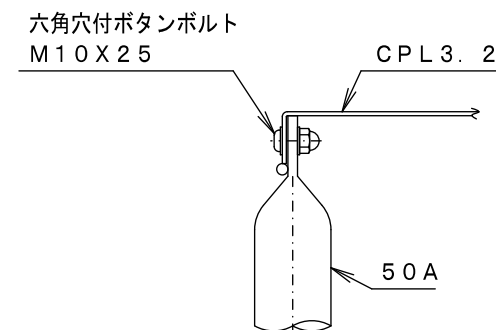
C詳細図 S=1/6
