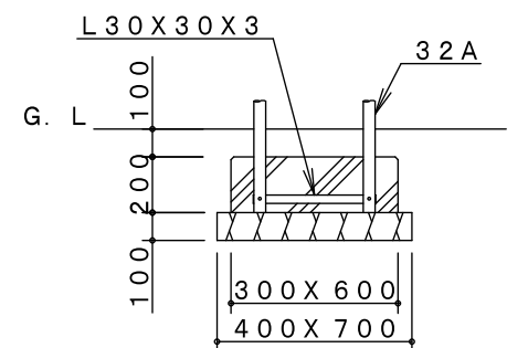
E基礎詳細図
