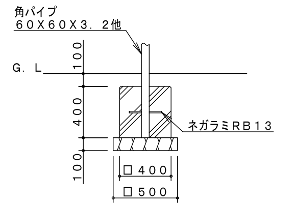
D基礎詳細図
