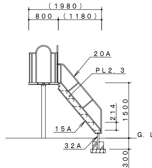
B-B' 矢視図
