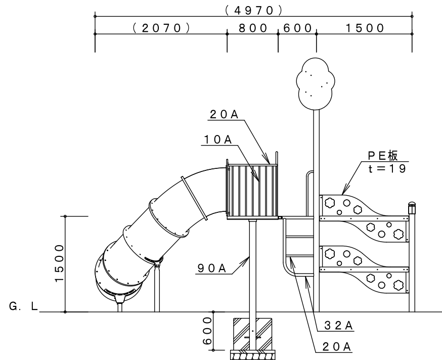
A-A' 矢視図
