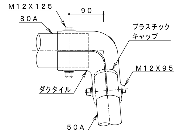
C詳細図 S=1/6
