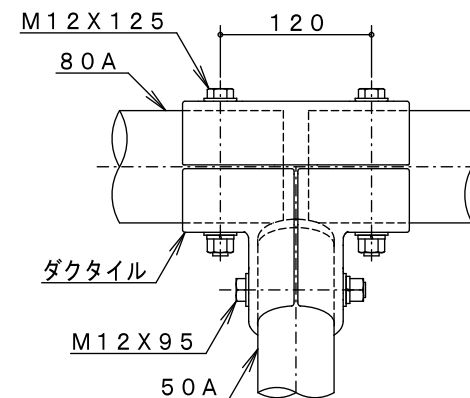
B詳細図 S=1/6
