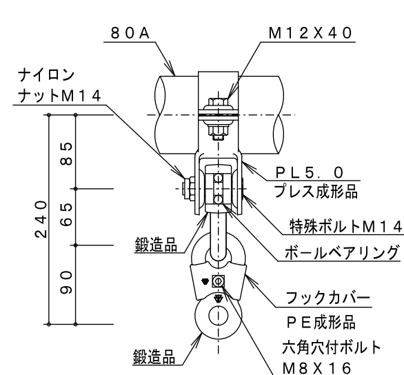
A詳細図 S=1/6
