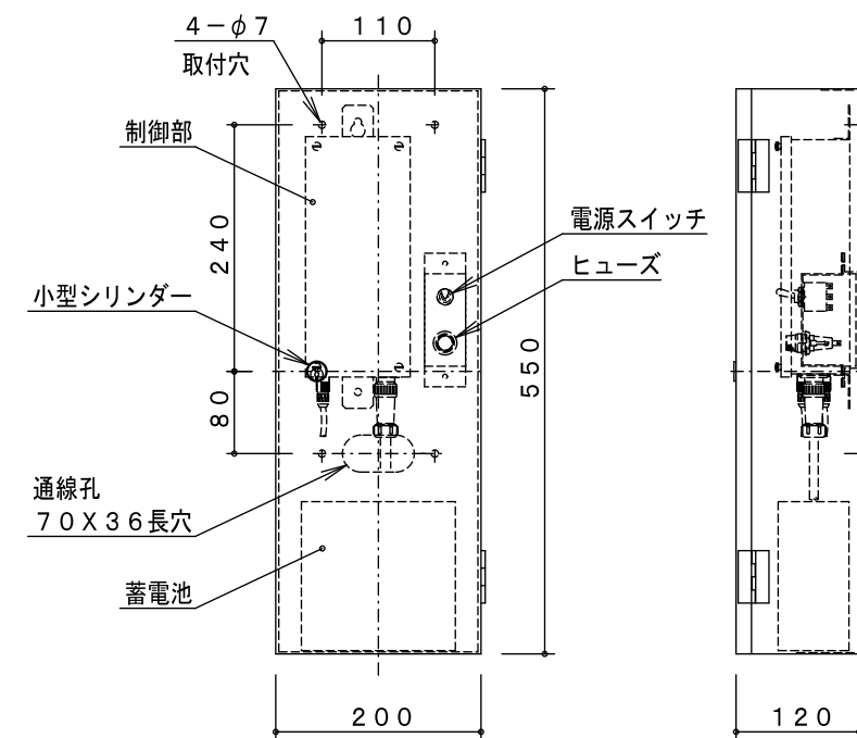
L E D 式内照太陽電池制御部詳細図 S = 1 / 8
