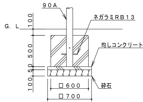
A基礎詳細図
