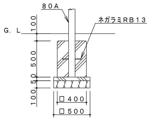
B基礎詳細図
