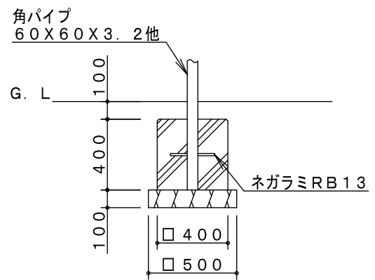
D基礎詳細図
