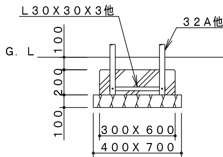
E基礎詳細図
