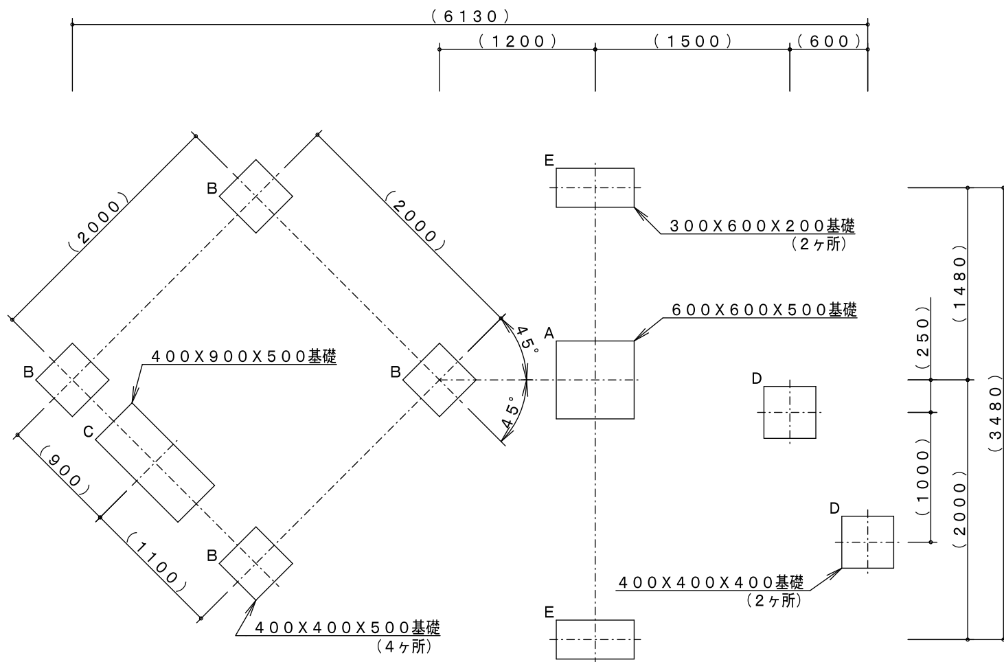
基礎平面図 S=1/40
