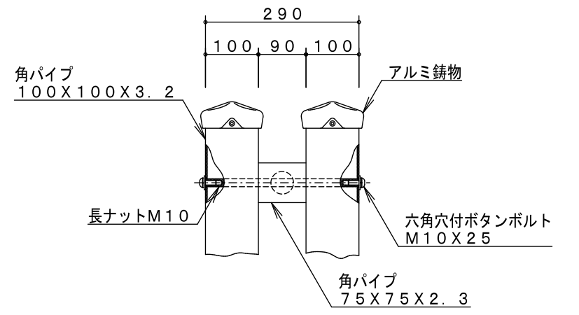
A詳細図 S=1/10
