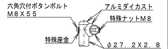
D詳細図 S=1/6
