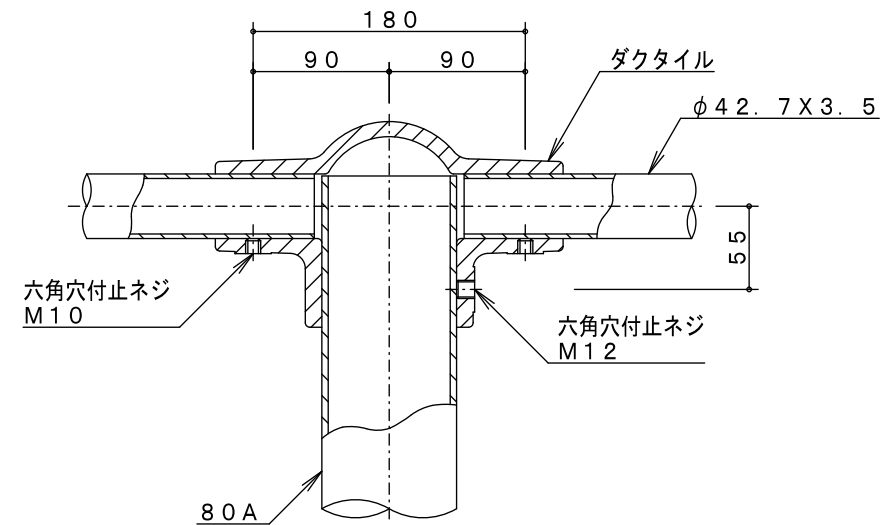
A 詳細図 S=1/5
