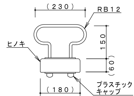
C詳細図 S=1/10
