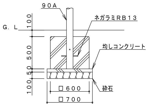
A 基礎詳細図
