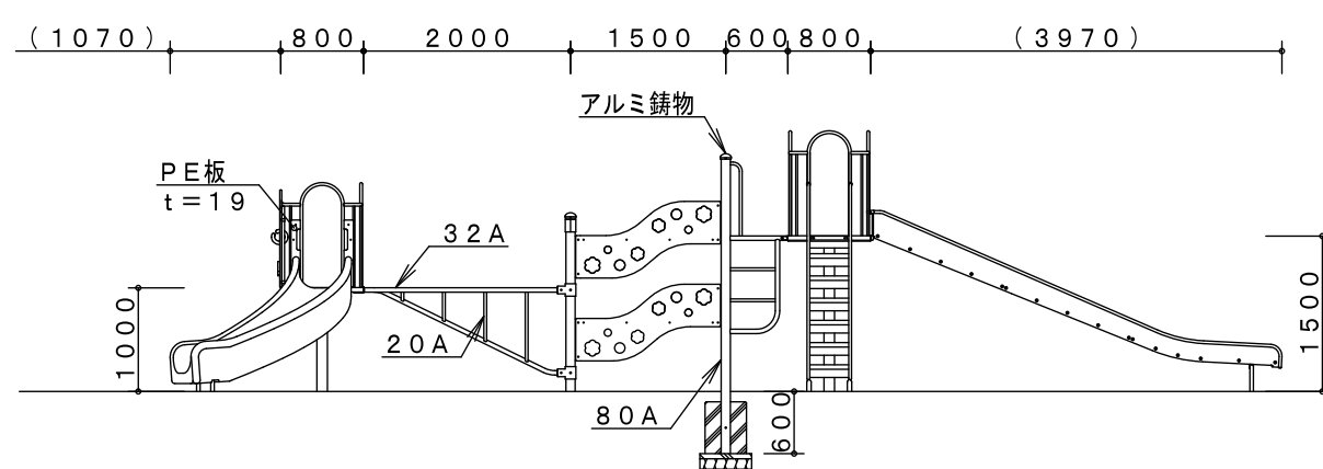
A-A' 展開図
