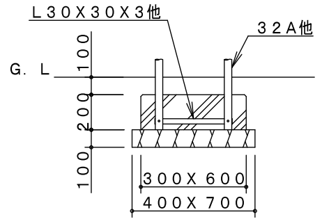
D 基礎詳細図
