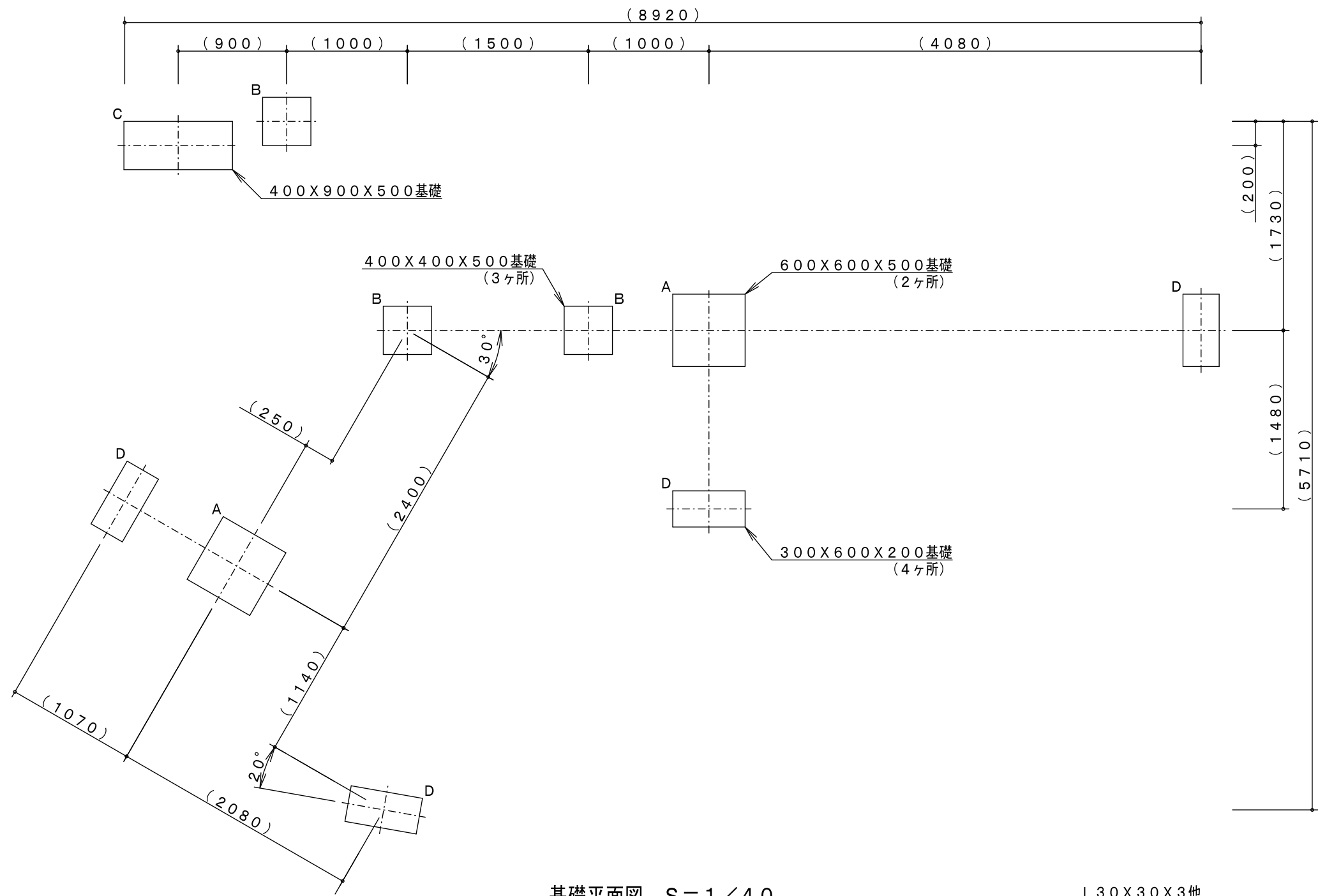
基礎平面図 S=1/40
