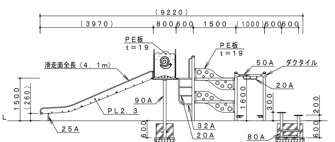
C-C' 矢視図
