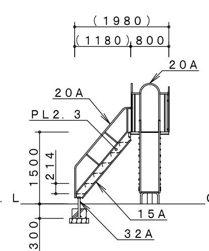
B-B' 矢視図
