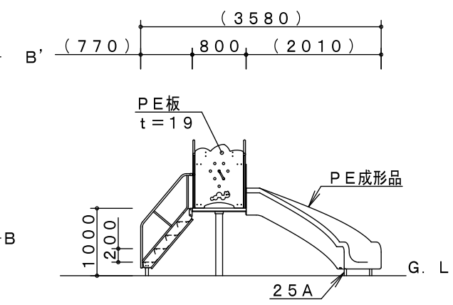
D-D' 矢視図
