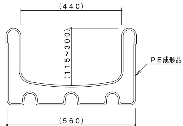
滑面断面図 S=1/10
