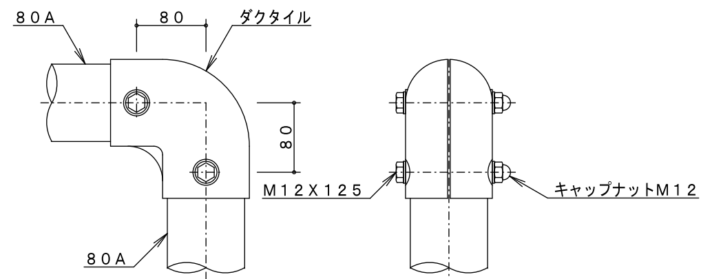
A詳細図 S=1/6
